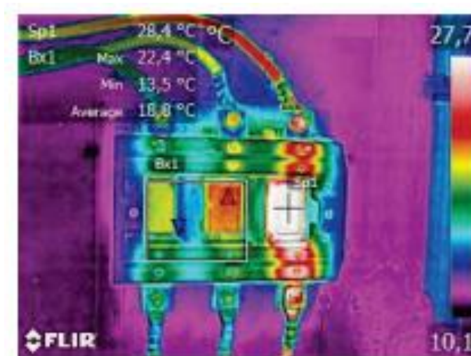
Slika 16. Pregrijavanje osigurača [23]
