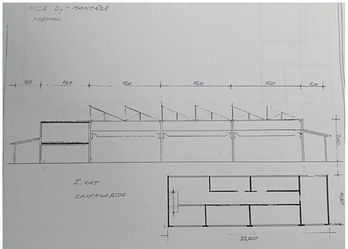
Slika 14. Hala D1-presjek [7]
