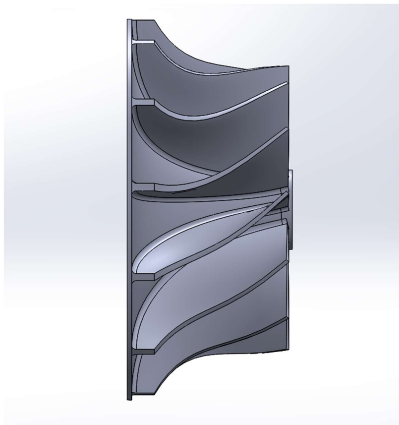
Slika 27: Rotor: pogled 1
