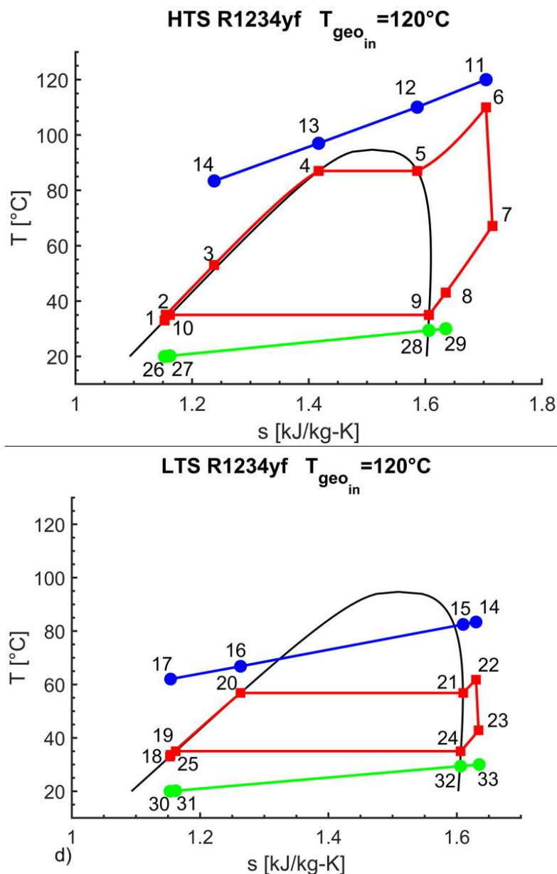
slika 7. T-s dijagrami
