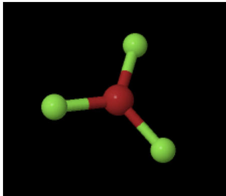
Slika 4: Prikaz molekule bromovog(III) – fluorida [11].
