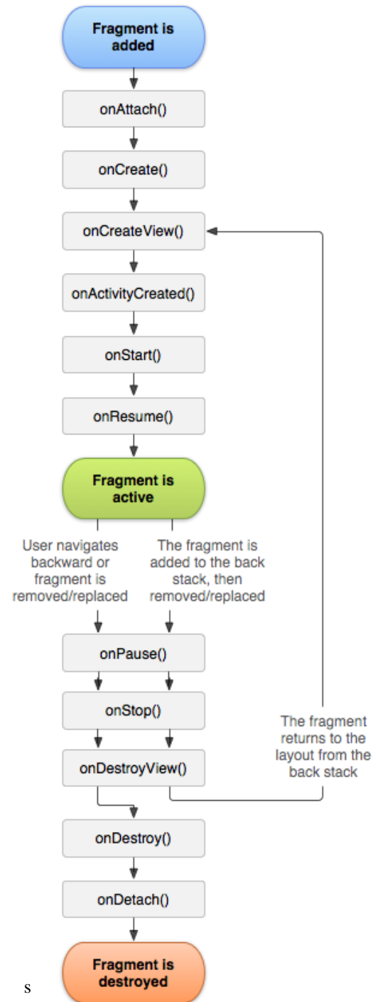
Slika 2.27. Grafička predodžba dijagrama životnog ciklusa fragmenta. (izvor: https://developer.android.com/guide/components/fragments.html )
