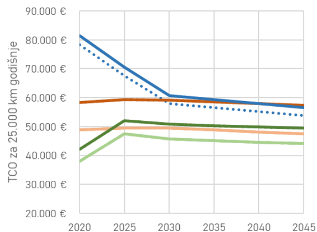
Cijena vodika +30%
