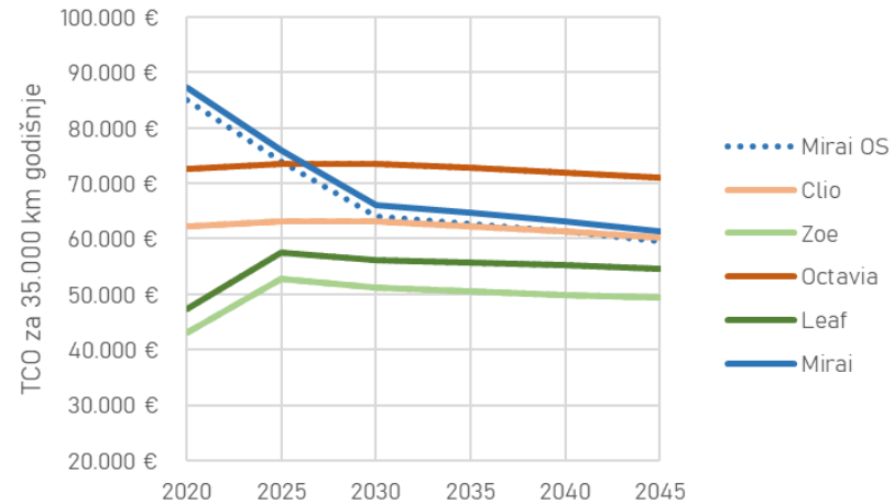
Cijena vodika +15%
