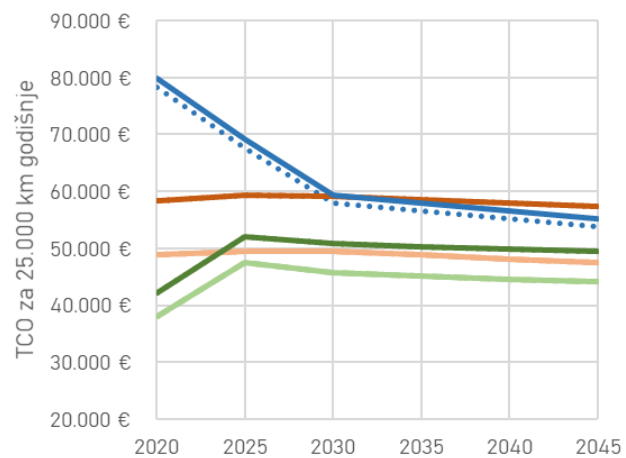
Cijena vodika +15%
