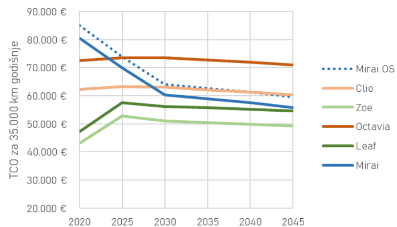
Cijena vodika -30%
