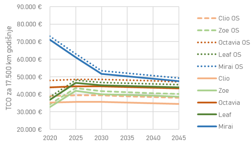
Diskontna stopa 7%
