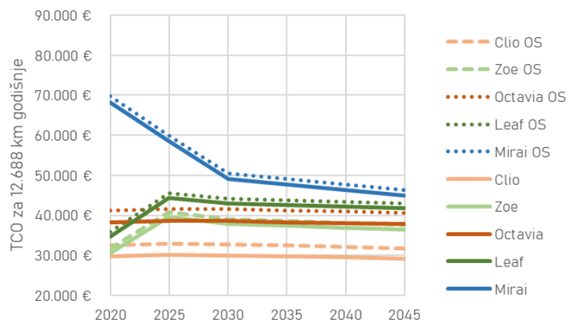
Diskontna stopa 7%
