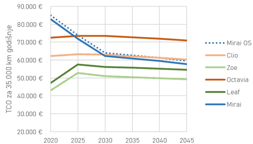
Cijena vodika -15%
